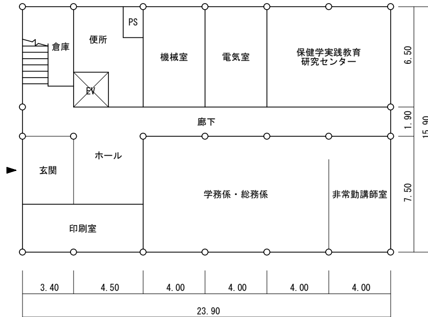
1 階平面図（改修前）S=1/250
